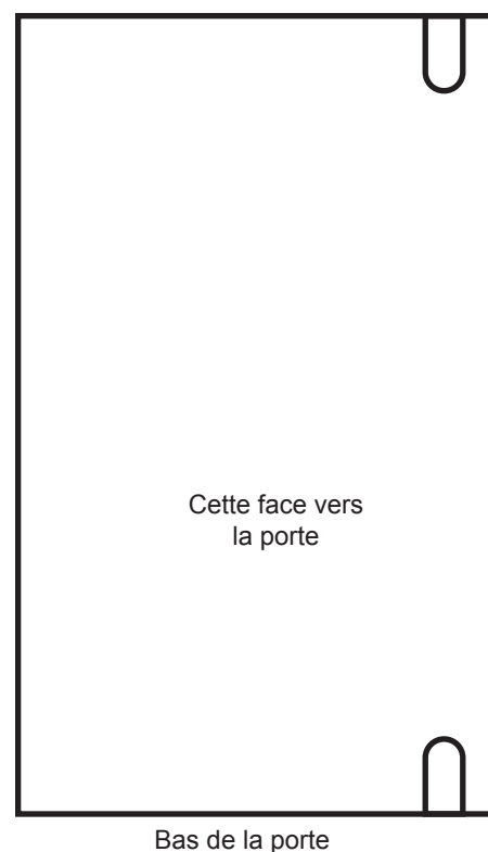
Figure 29 Dimensions de panneau pour porte à charnières à gauche
